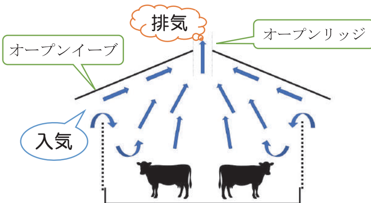
図1. 温度差を利用した換気
